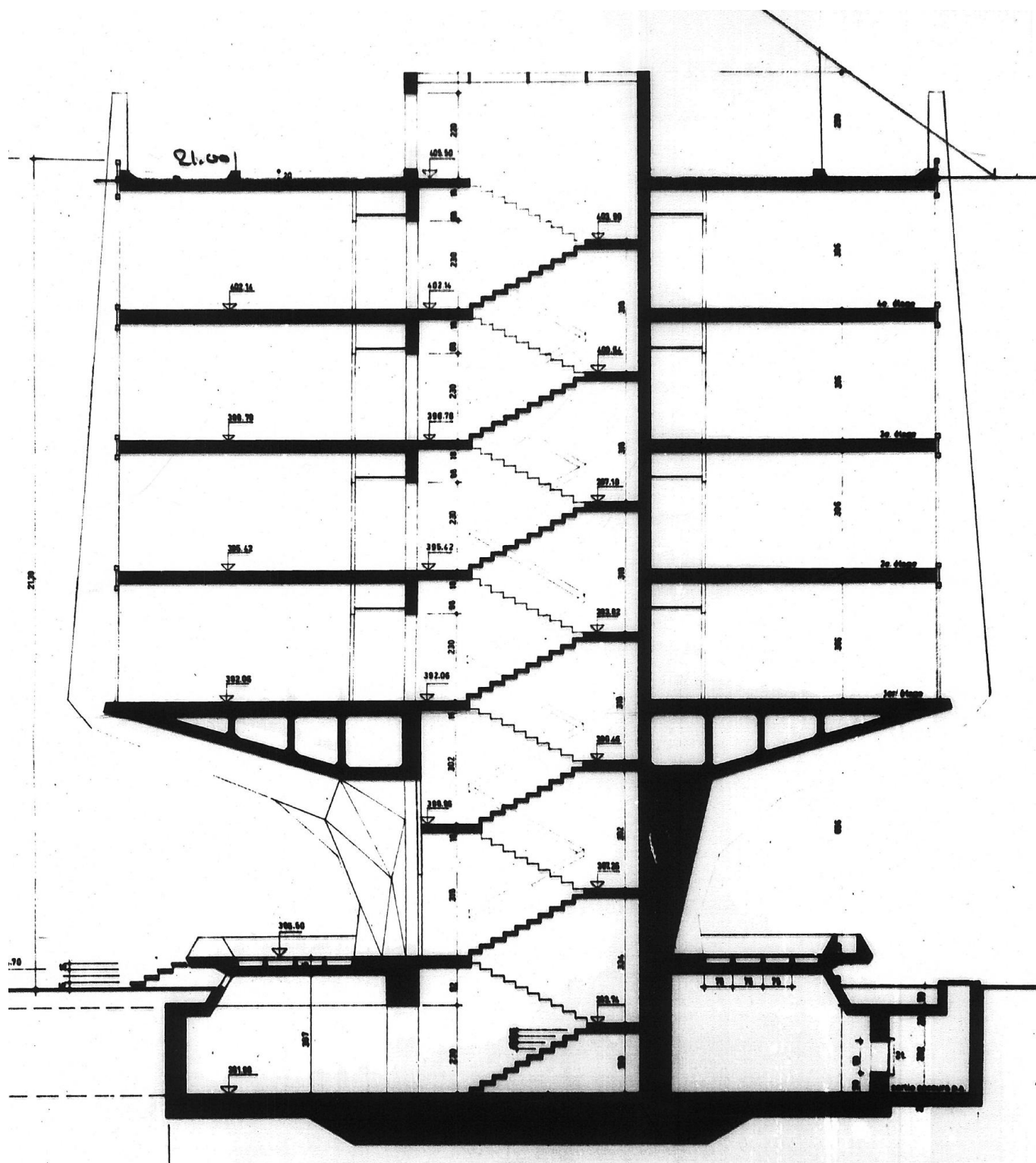
"Тюльпан" в разрезе - план здания © Jack Bertoli
