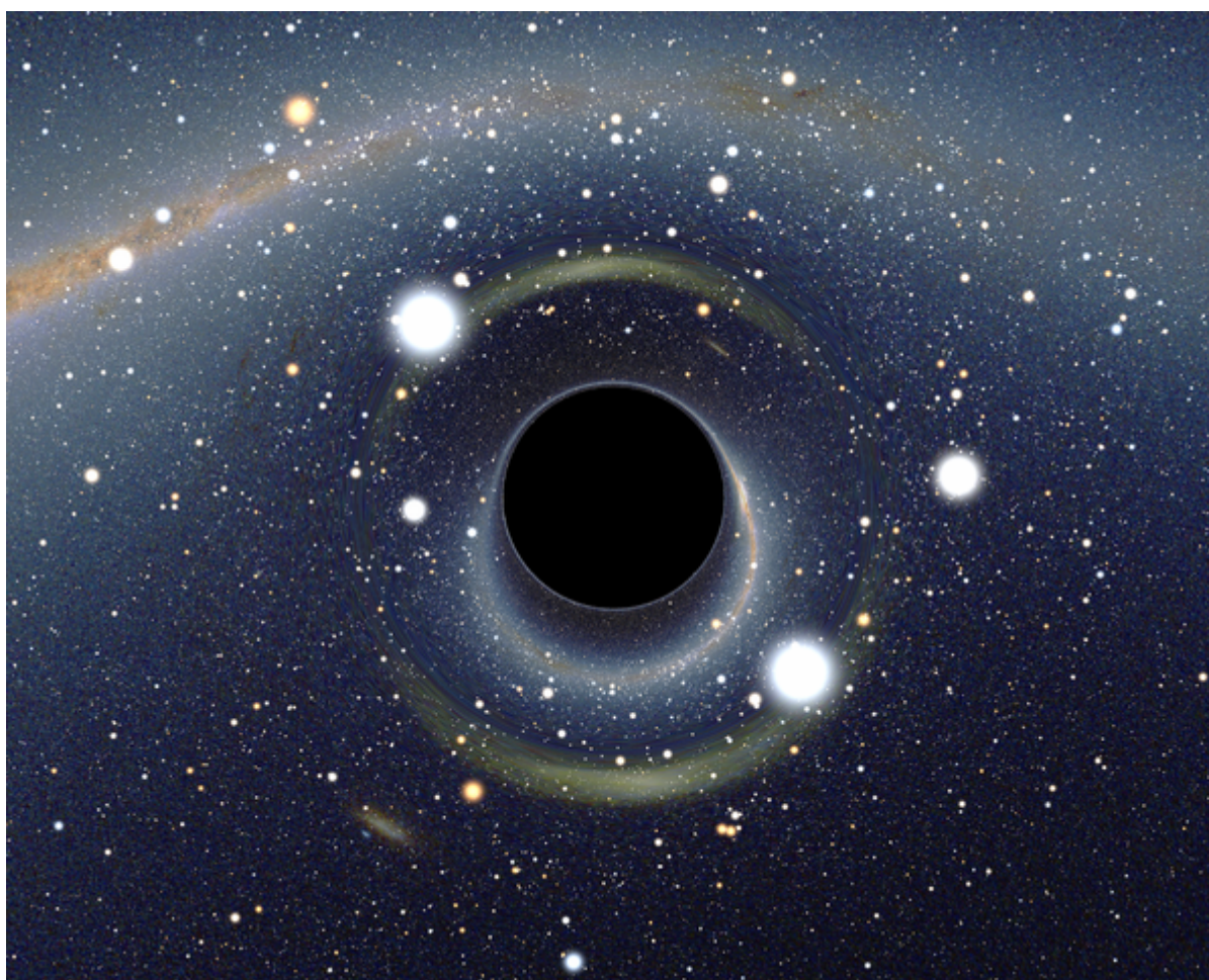
Модель черной дыры вблизи Туманности Магеллана ЦЕРН
